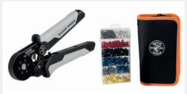
Juego de Ponchadora Hexagonal para Ferrules 34061
